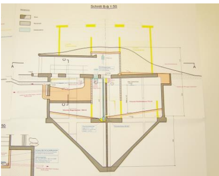
Projektplan für den Umbau der ARA
